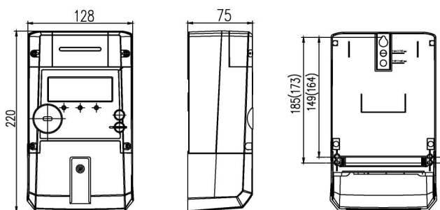
Dimension (Unit:mm)
